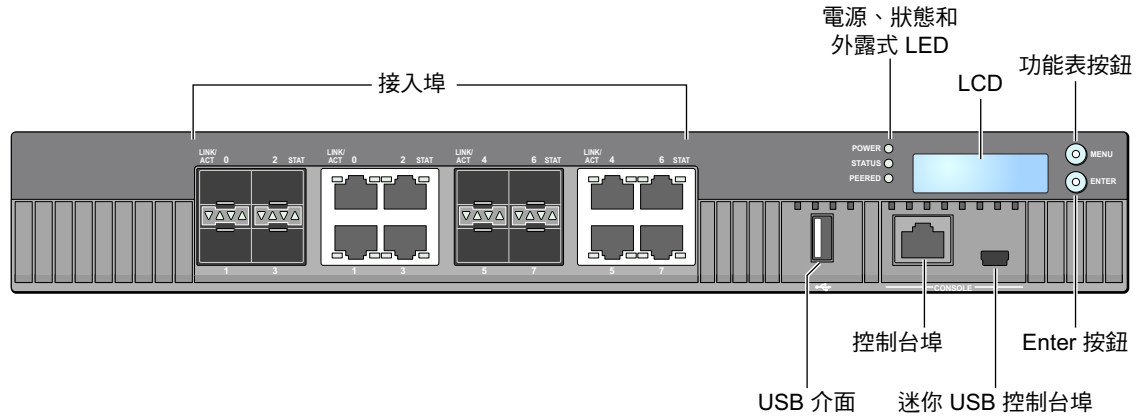
圖 1 W-7030 控制器的前置面板
