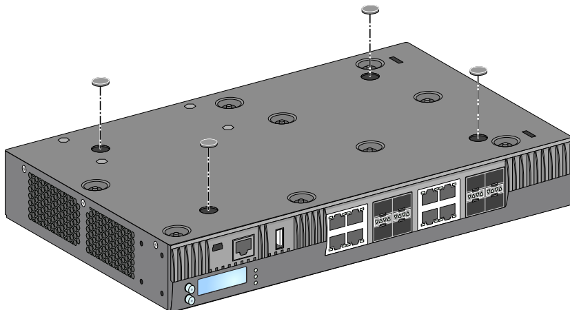
圖 9 連接橡膠腳墊
