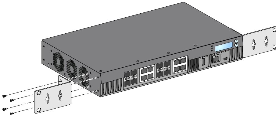
圖 7 機架安裝托架
