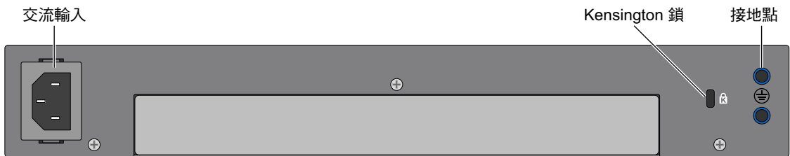
圖 2 W-7030 控制器的後置面板
