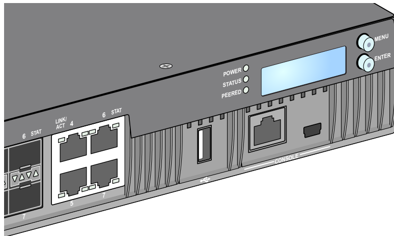
圖 4 埠、LED 和 LCD 面板
