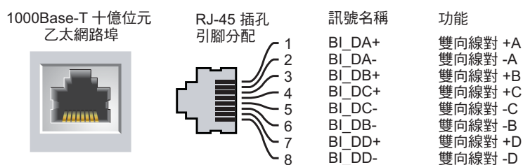
圖 3 10/100/1000BASE-T 管理埠引出線
