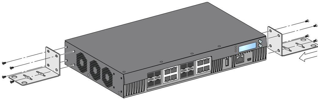
圖 10 安裝壁式安裝托架
